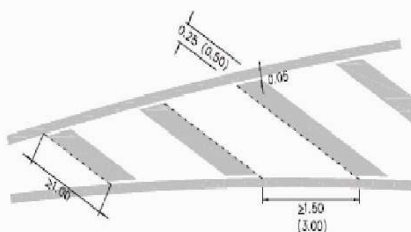
Σχήμα Η2-1: Λεπτομέρεια επιφάνειας αποκλεισμού
