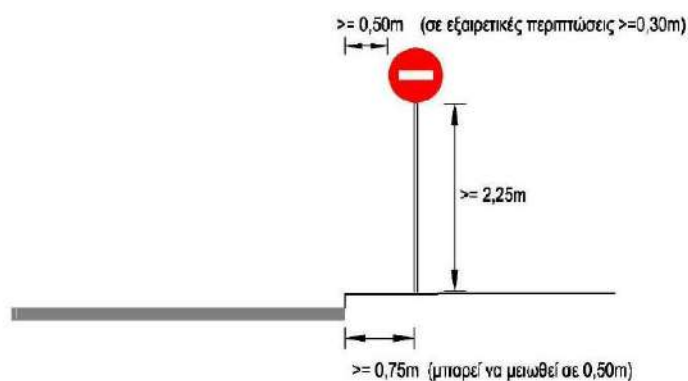
Σχήμα 2. Τοποθέτηση πινακίδων στον ιστό του σηματοδότη
