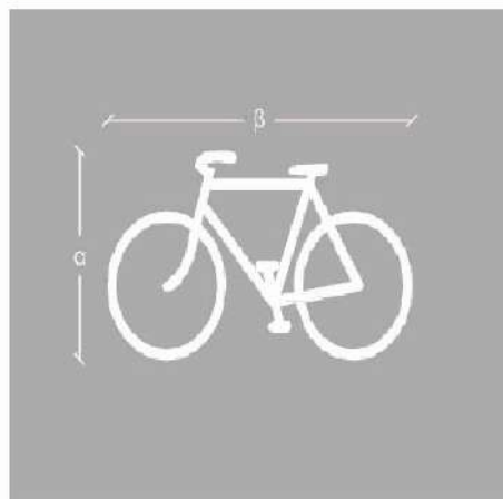
Σχήμα 0-7 Σύμβολο ποδηλάτου
