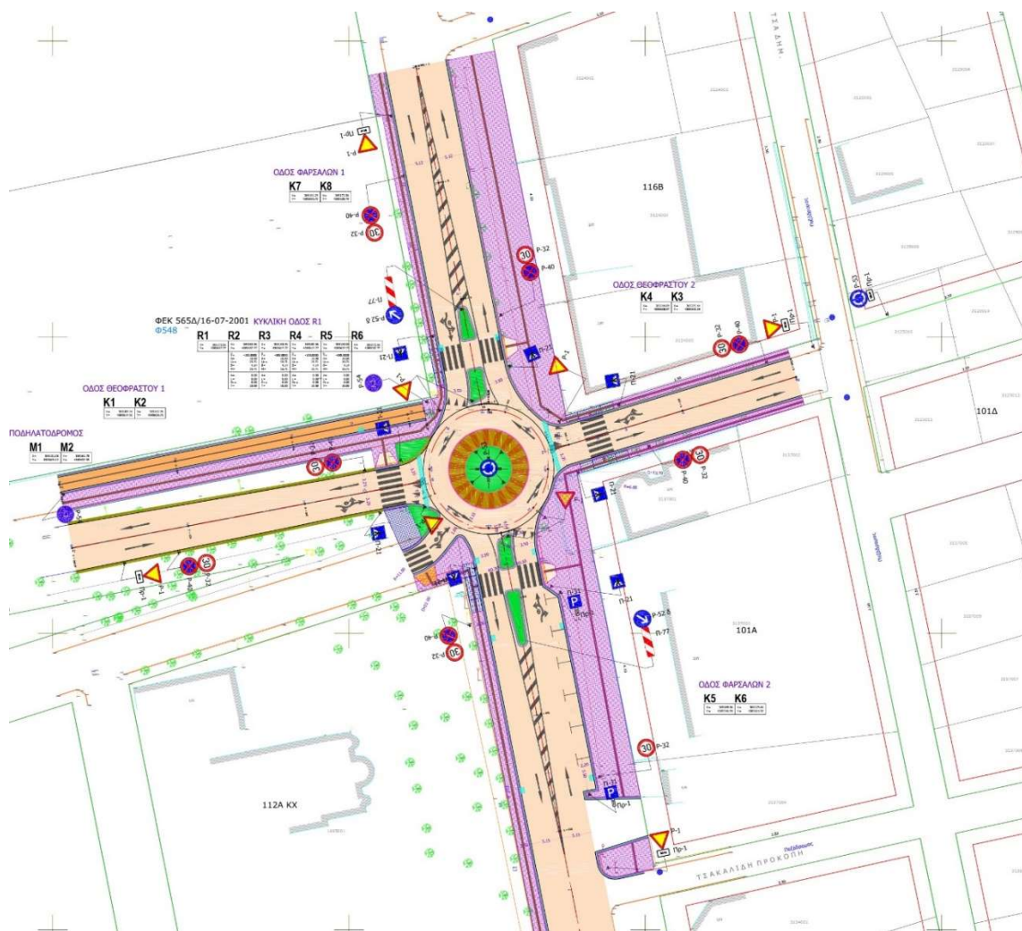
Εικόνα 6.Οριζοντιογραφική αποτύπωση Κ3 (Ιδία επεξεργασία)
